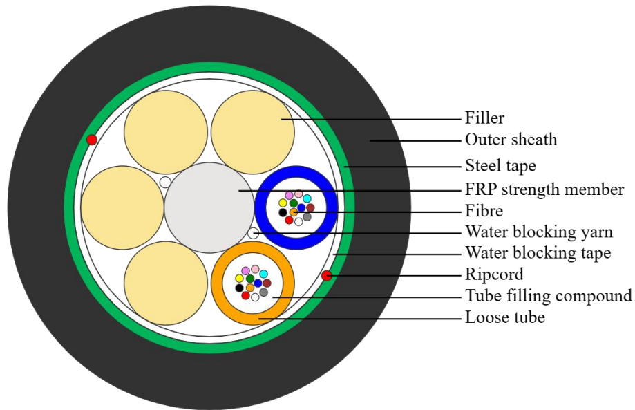
GYFS-240M4
